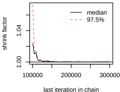
d.Icotinib.Befotertinib
