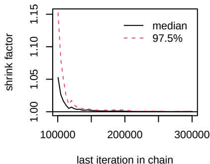
d.Erlotinib.DHFRi
