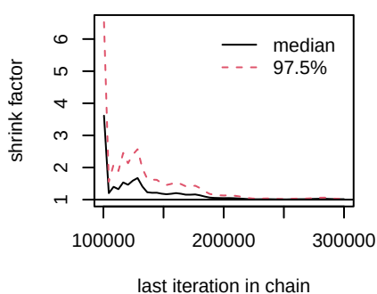
d.Gefitinib.Icotinib
