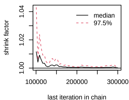
d.Gefitinib.Lazertinib
