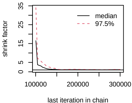
d.Gefitinib.Gefitinib_PARPi
