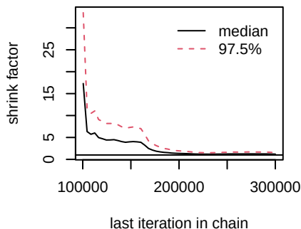
d.Osimertinib.chemo_antiangio
