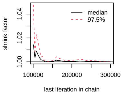
d.Gefitinib.Furmonertinib
